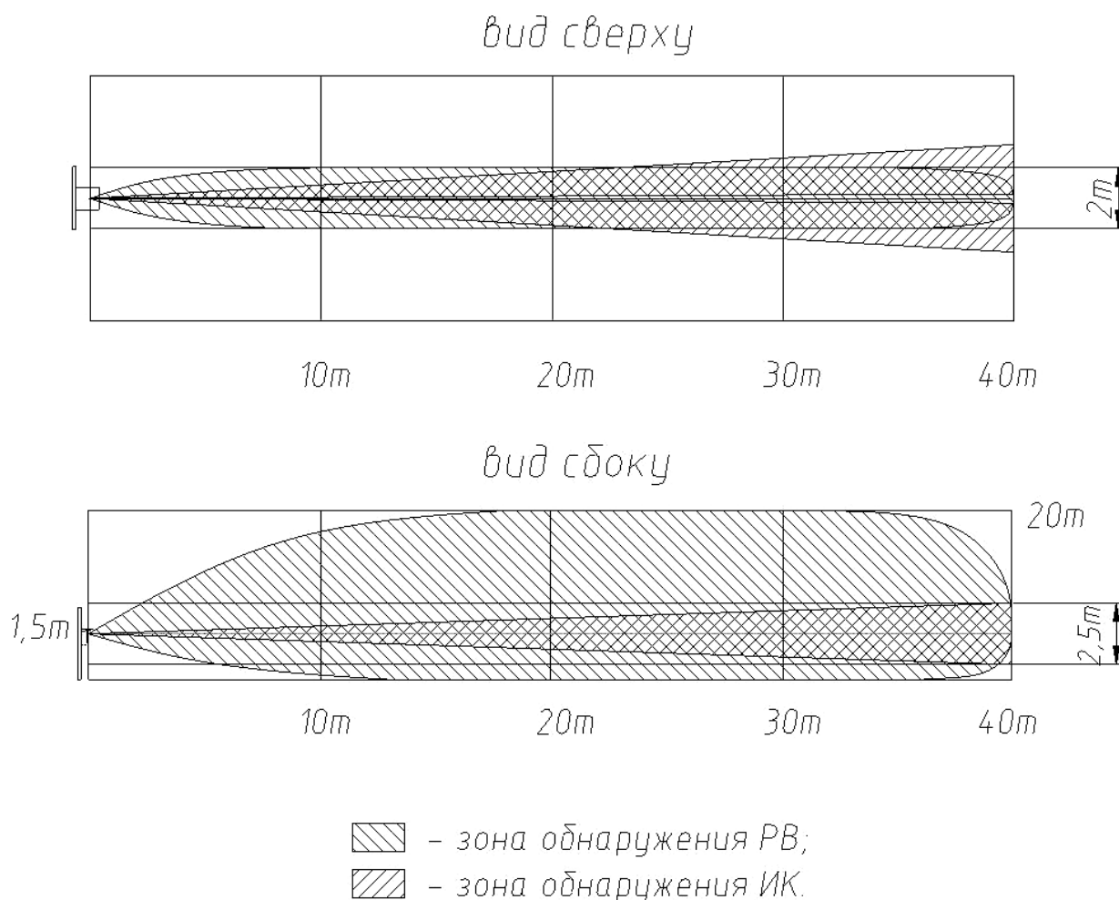
Рисунок 3.1 – Размеры зоны обнаружения извещателя «Циклоп-30»
