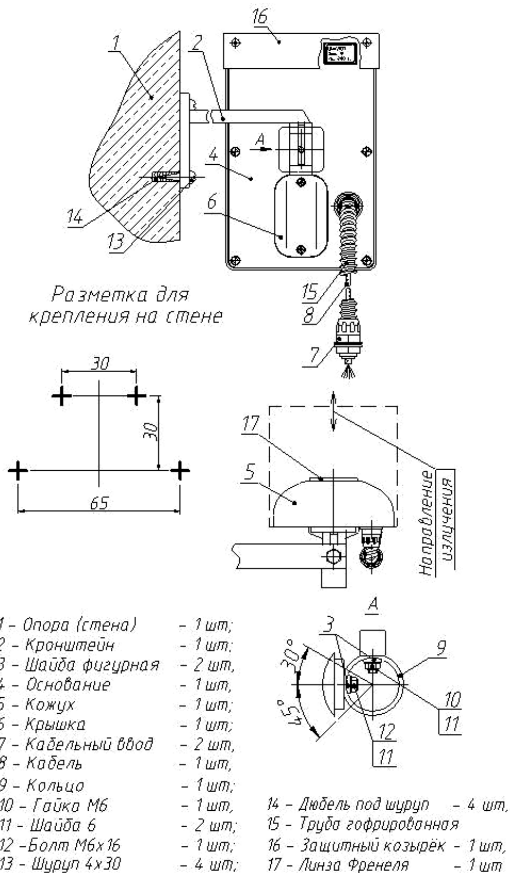
Рисунок 6.2 – Установка извещателя на стене.
